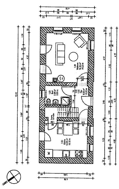
Grundriss ERDGESCHOSS
