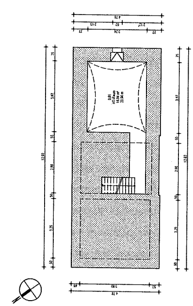
Grundriss KELLERGESCHOSS
